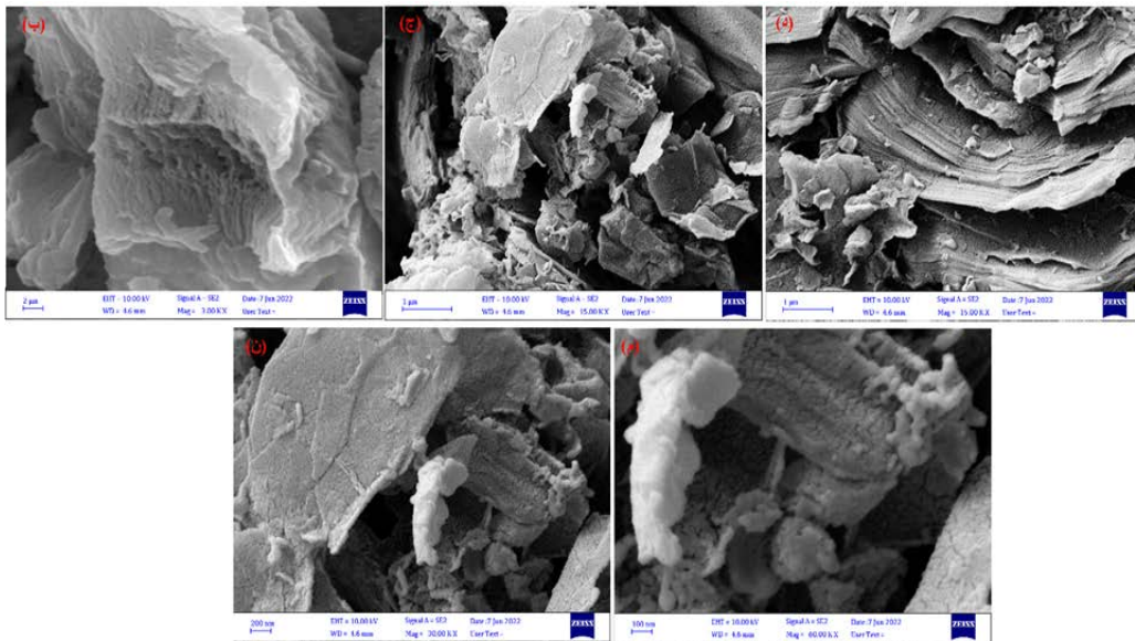
شکل ۱: ترموگرام (الف) و میکروگراف های نانوجاذب سنتز شده با بزرگنمایی های مختلف (ب-م)
