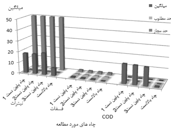
نمودار ۳: میانگین نیترات و فسفات و COD در چاه‌های مورد مطالعه و مقایسه با استانداردهای ملی آب آشامیدنی (بر حسب \text{mg}/\text{l} )
