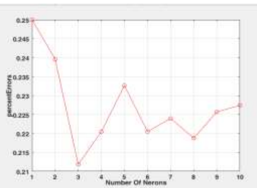
شکل ۲- الف. خطای معماری‌های مختلف شبکه MLP به ازای تغییرات تعداد نرون در لایه مخفی
