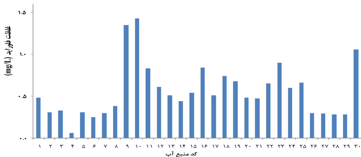
شکل ۲- غلظت فلورايد در منابع مورد مطالعه برحسب میلی‌گرم بر لیتر
