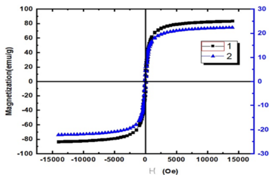
شکل ۵: خواص مغناطیسی نانوذرات سنتز شده (۱) نمونه \text{Fe}_3\text{O}_4 و (۲) نمونه \text{Fe-doped TiO}_2 @ \text{Fe}_3\text{O}_4
