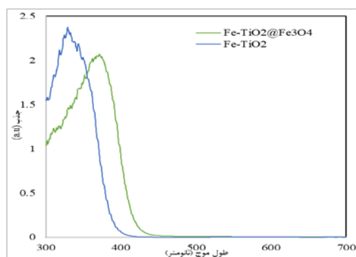
شکل ۴: طیف جذب نور مرئی - طیف فرابنفش (DRS) نمونه های \text{Fe-doped TiO}_2 @ \text{Fe}_3\text{O}_4 و \text{Fe-doped TiO}_2
