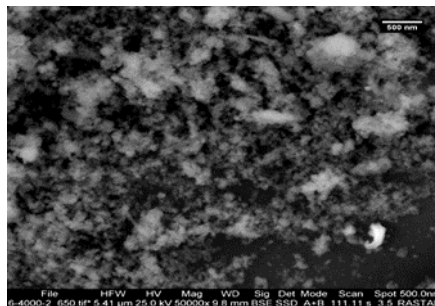
شکل ۱: تصویر SEM نانوذرات Fe-doped TiO 2 @Fe 3 O 4
