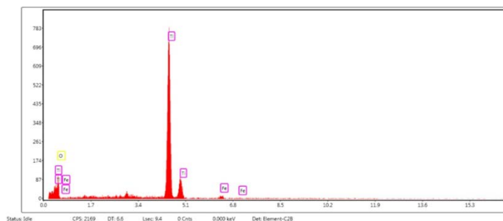
شکل ۲: طیف EDX برای ذرات Fe-doped TiO 2 @Fe 3 O 4
