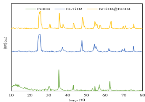
شکل ۳: طیف XRD نانوذرات \text{Fe}_3\text{O}_4 ، \text{Fe-doped TiO}_2 و \text{Fe-doped TiO}_2 @ \text{Fe}_3\text{O}_4
